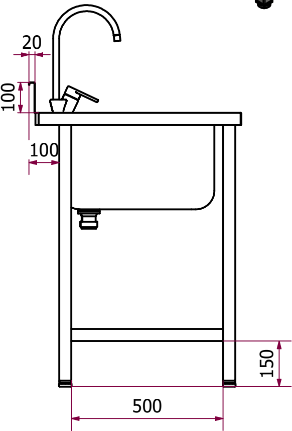
VISTA LATERAL
