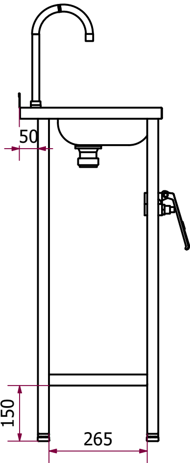
VISTA LATERAL
