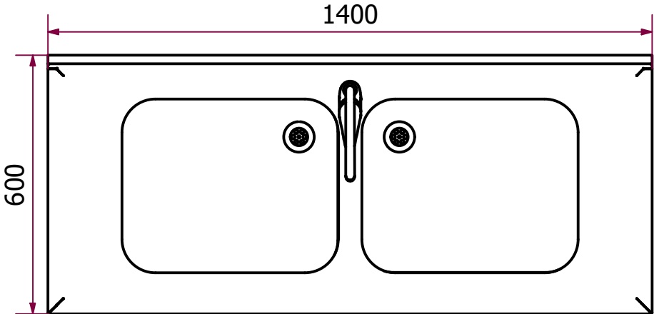
VISTA SUPERIOR
