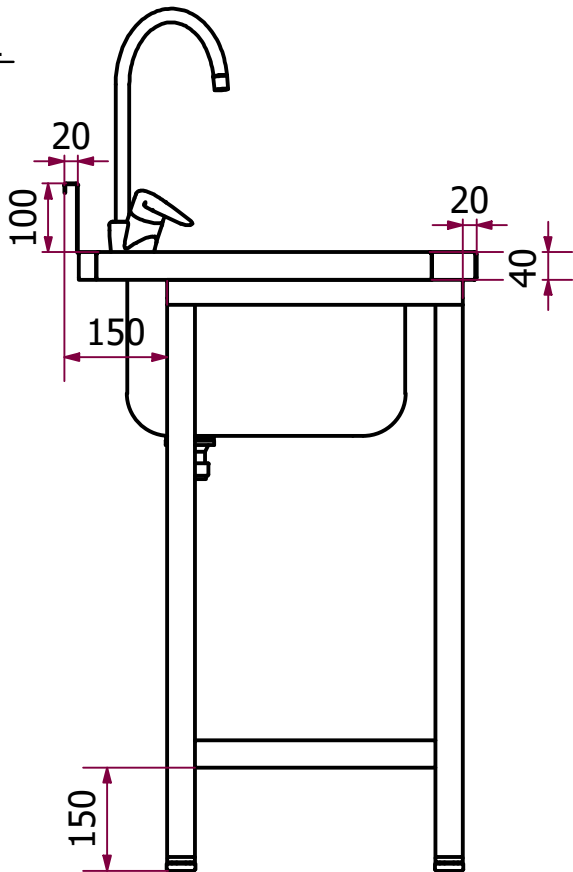
VISTA LATERAL
