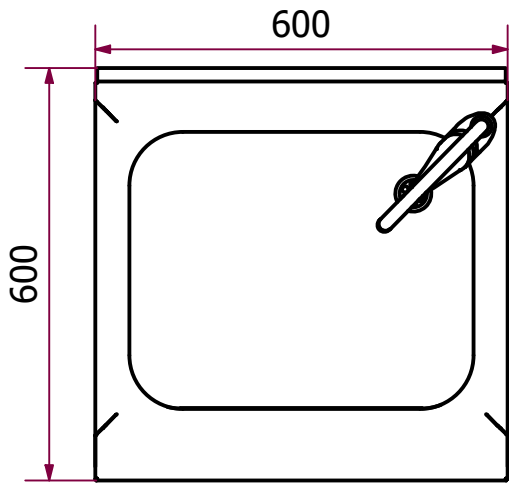
VISTA SUPERIOR
