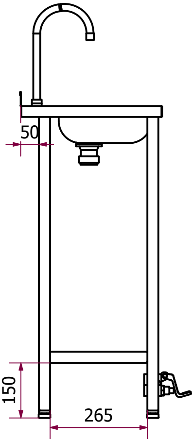
VISTA LATERAL
