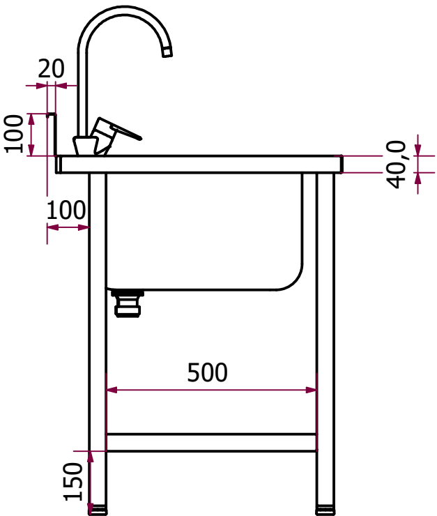
VISTA LATERAL
